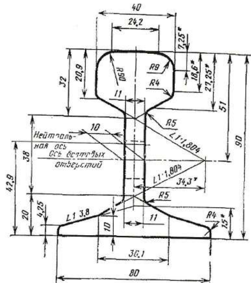
Рис. 2 Рельс Р18
