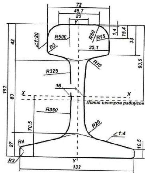
Рис.1 Рельс Р 50
